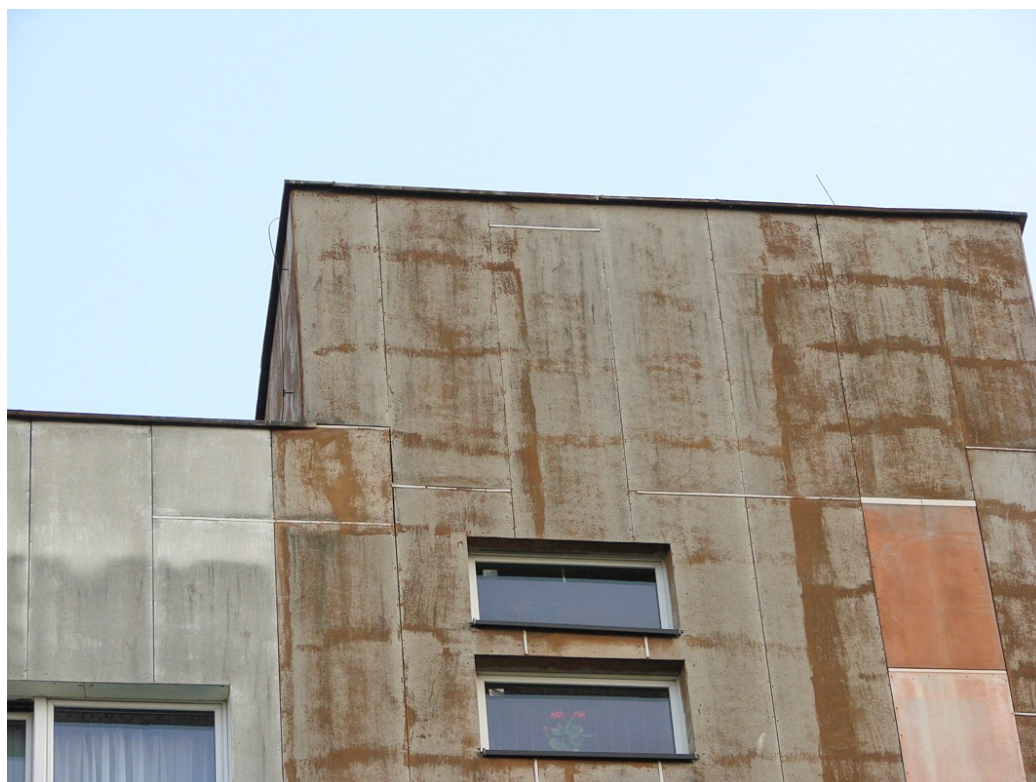
Fot.10. Widok części stropowej budynku od strony północnej (aut. Szymon Wójcik)
