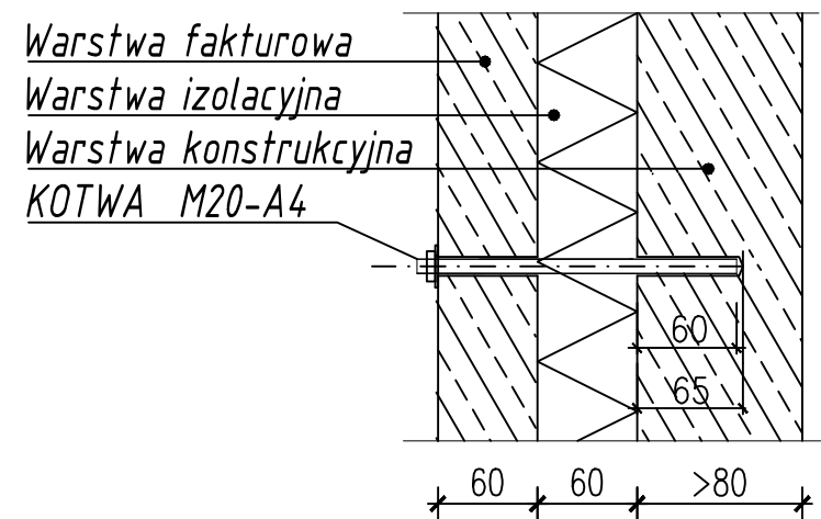
Przekrój pionowy 1:5
